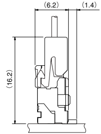
PAF Receptacle + PA Header
