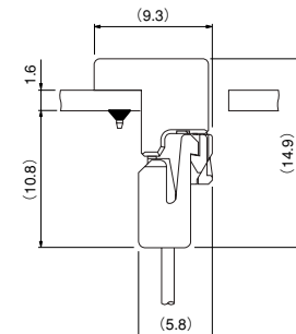
PAF Receptacle + PA bottom type header
